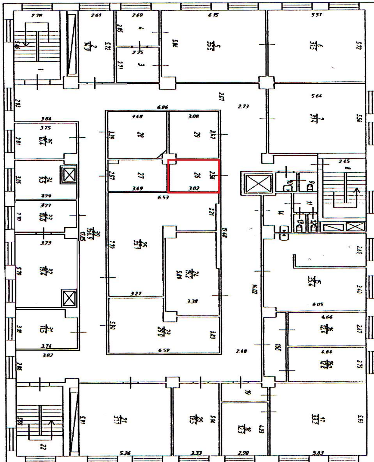
План 2 этажа
