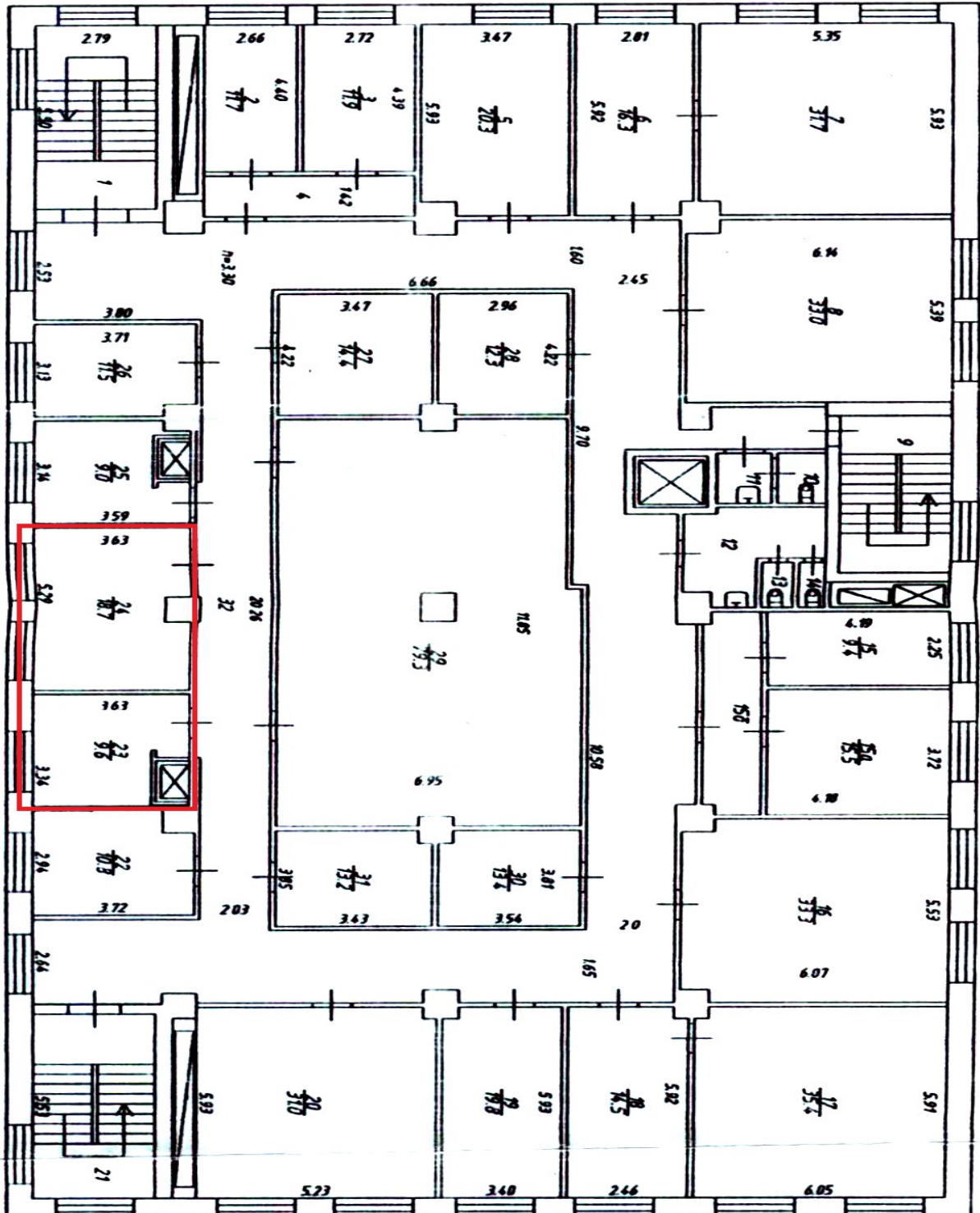
План 3 этажа
