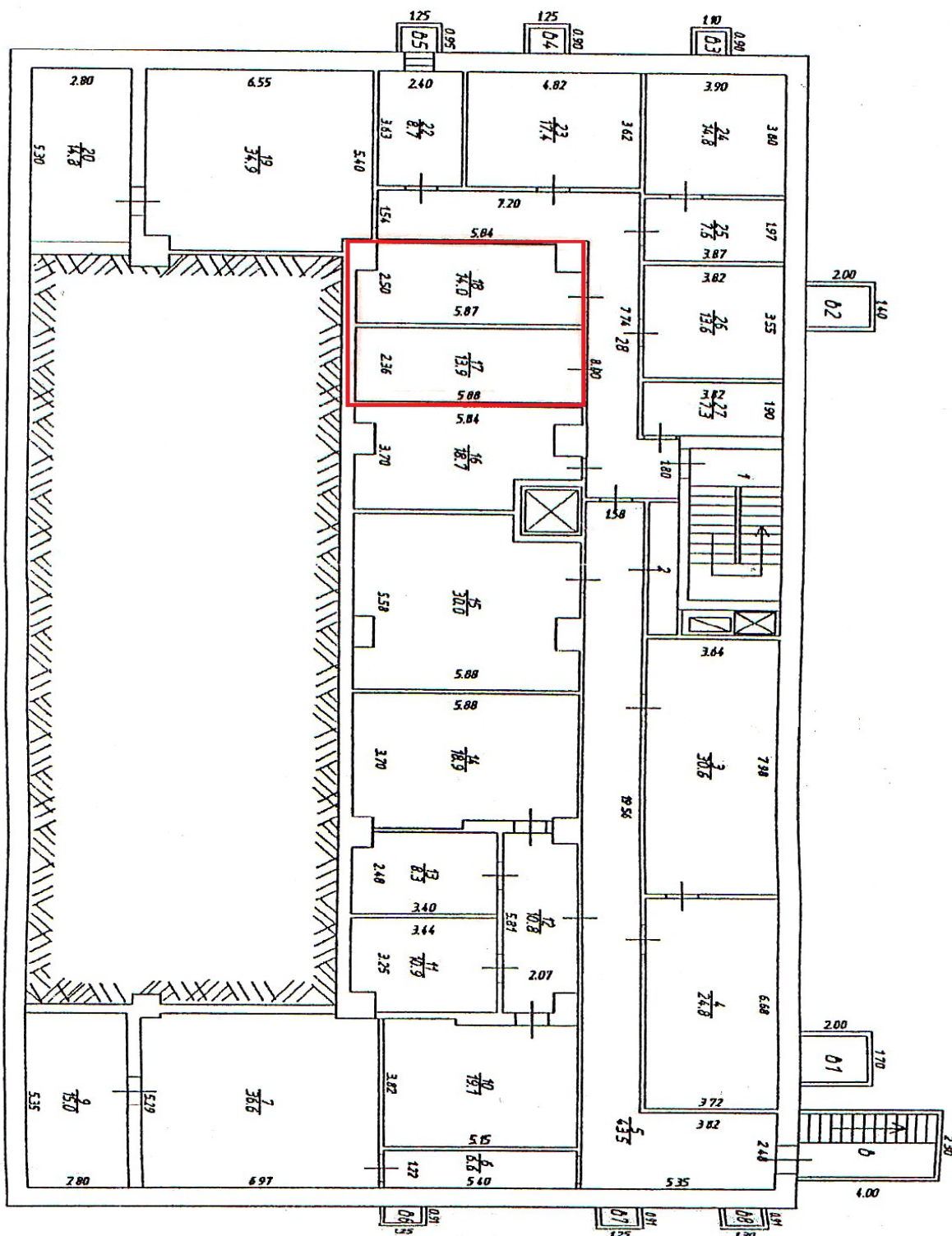
План подвала
